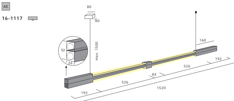
4 x T16 · G5 · 230V · 24W · EVG
