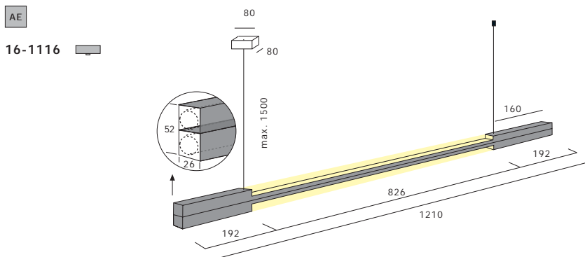
2 x T16 · G5 · 230V · 21W · EVG
